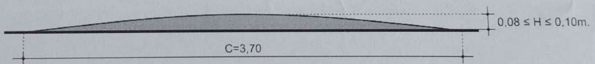
CORTE A-A
